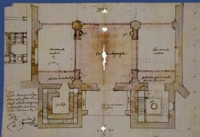
Trazas del pórtico y coro realizadas por Juan Gómez de Mora en 1639.
