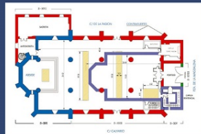
Plano comparativo de las dos iglesias -la Vieja y la Nueva- (José M o Real y Martín Sánchez)
